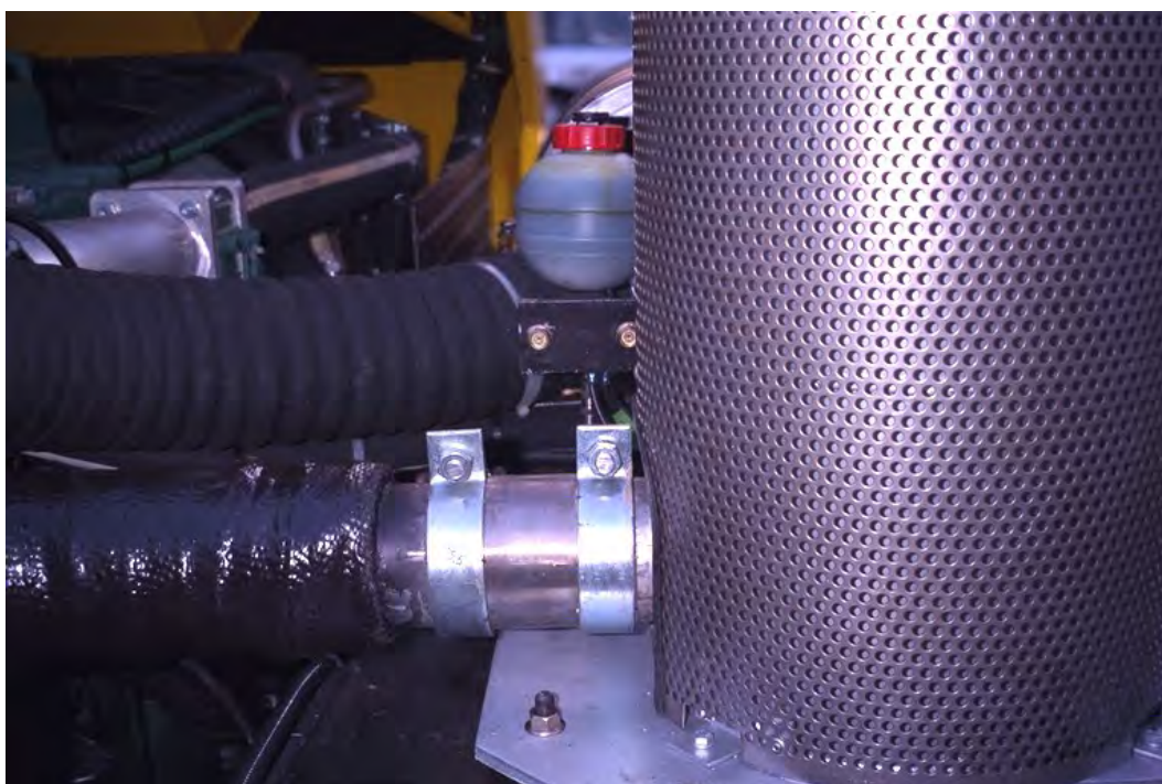
Anschluß am DPF mit 2 Rohrschellen (ohne Handschutz)
