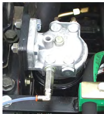
Rückschlagventil wird in den Kraftstofffilter eingeschraubt
