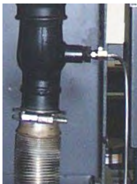
Revisionsstutzen für Abgasmessung vor dem Filter
