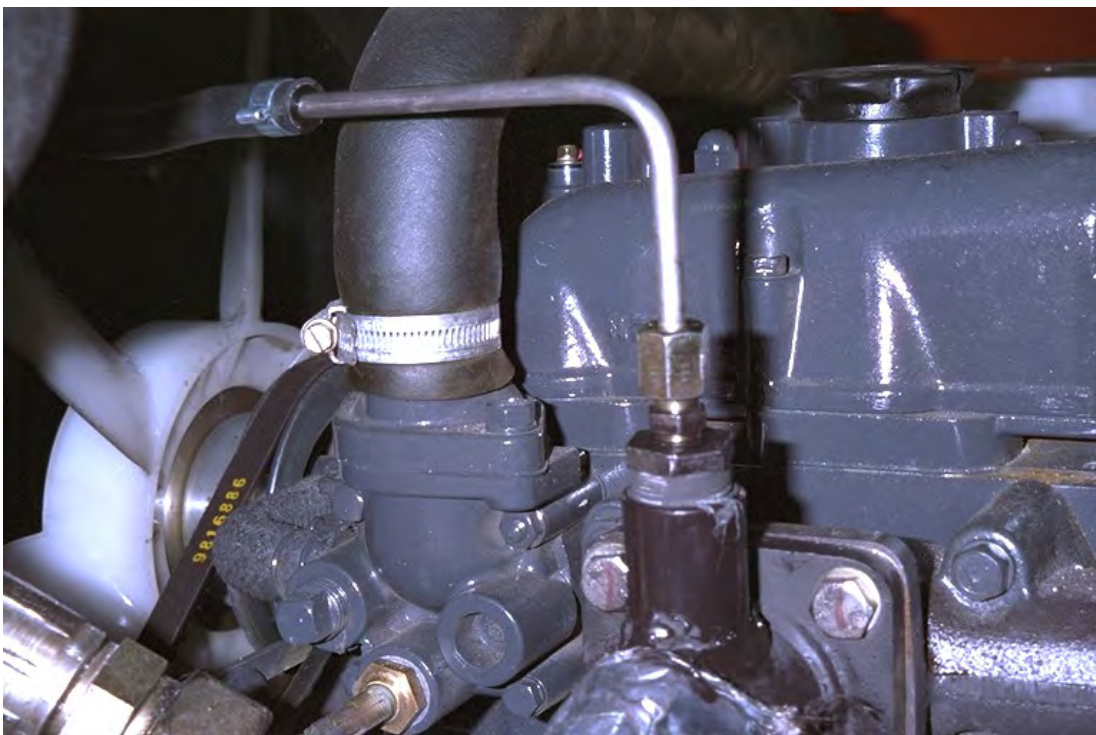
Revisionsstutzen mit Ausgang für Abgasgedrucktüberwachung.
